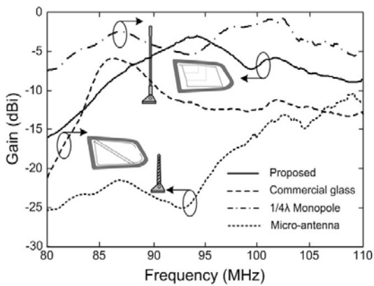
그림 8. 투명도가 향상된 안테나의 전방향 이득
